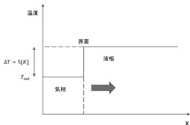
図 2 ステファン問題の温度分布
