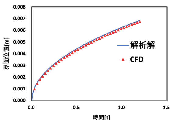
図 3 界面位置の解析解との比較
